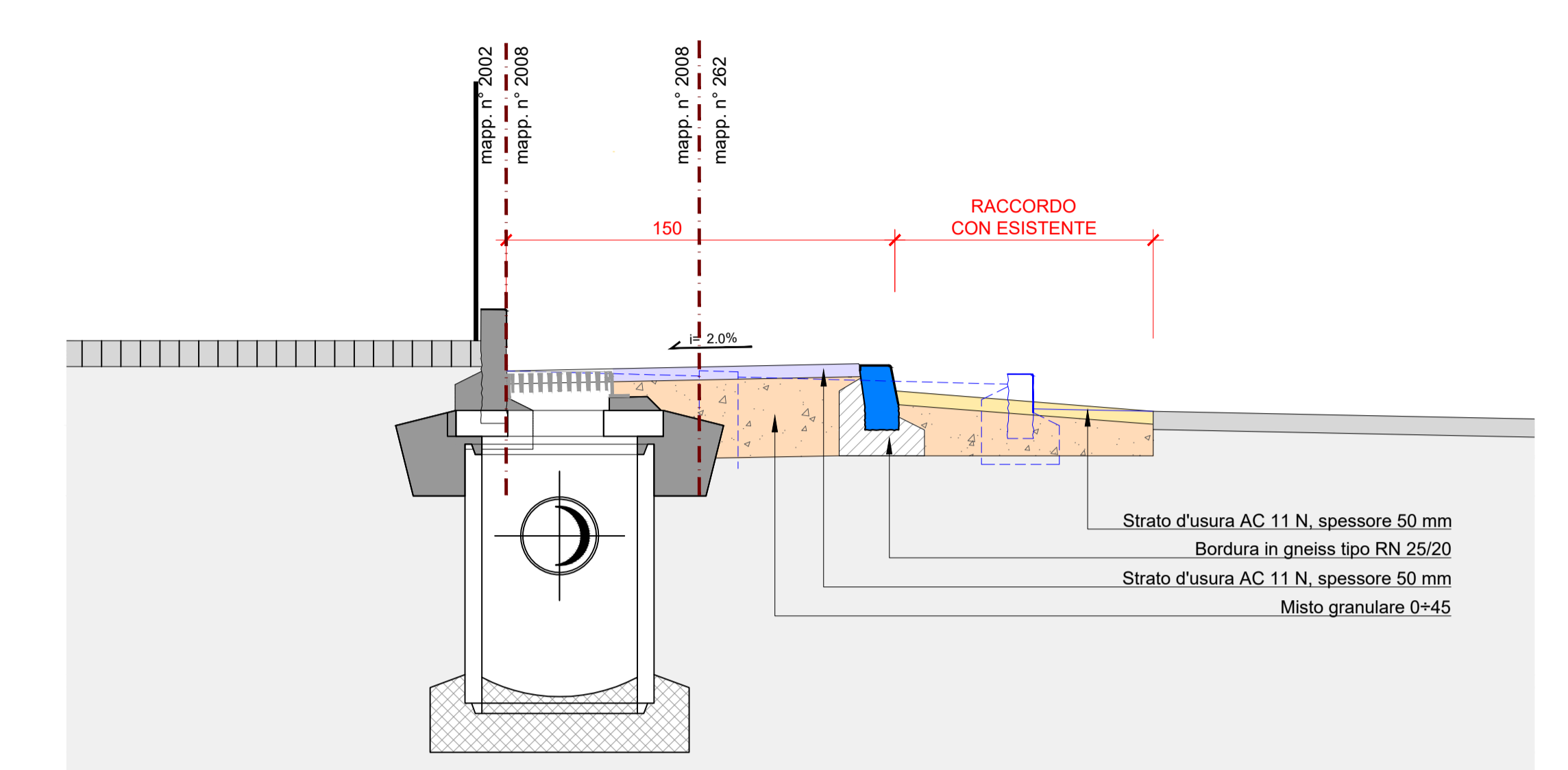
Sezione A-A 1:20
