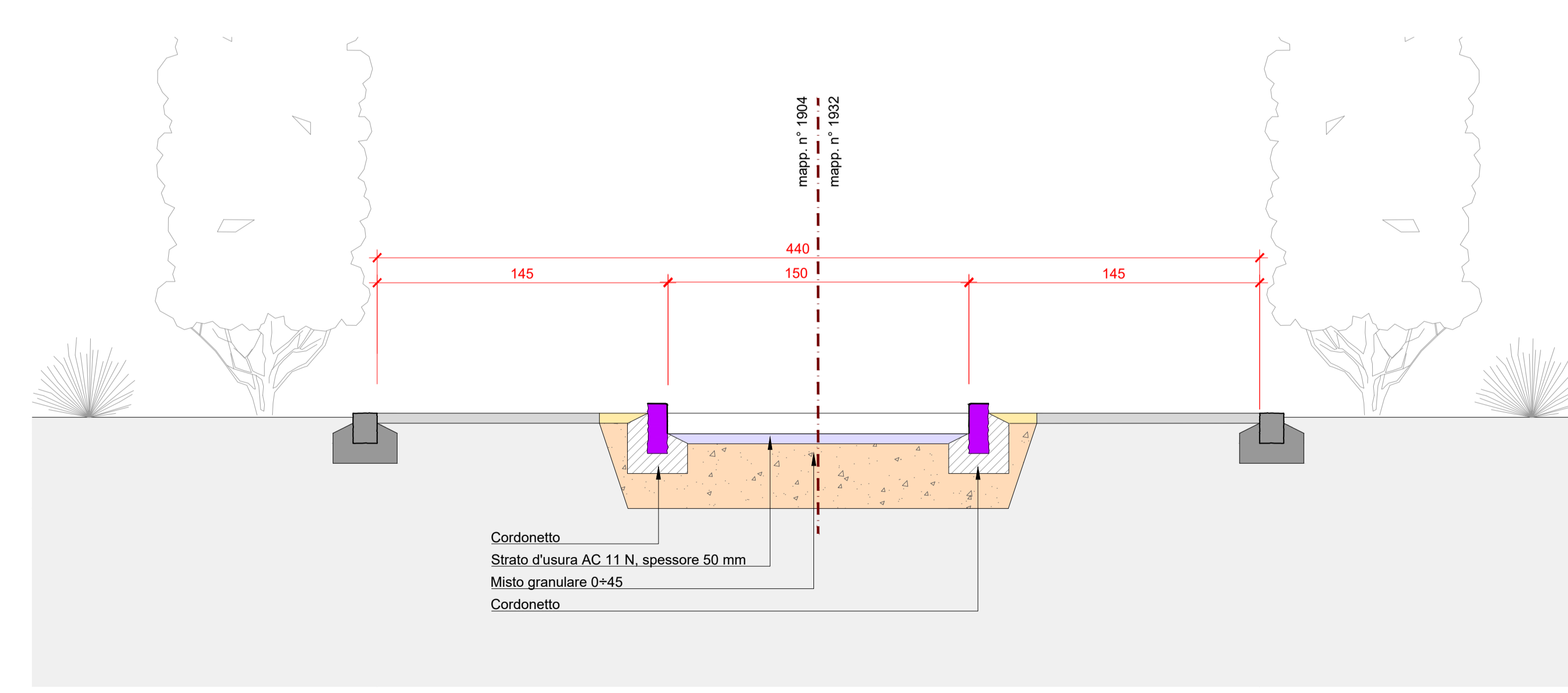
Sezione B-B 1:20
